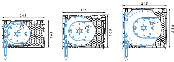
Coffre de 235 BLOC BAIE XXL dédié à la lame BIO et RS52
