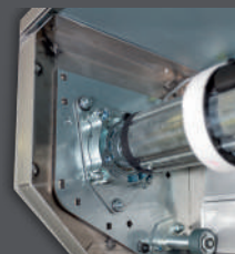
Joue acier sur silent-bloc Roulette souple anti-bruit
